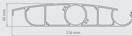
Sezione dell'aletta
