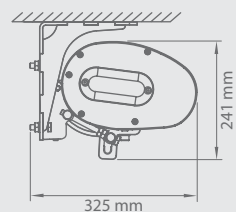
Montaggio a soffitto
