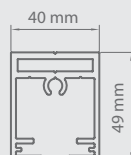
Sezione del telaio laterale e inferiore
