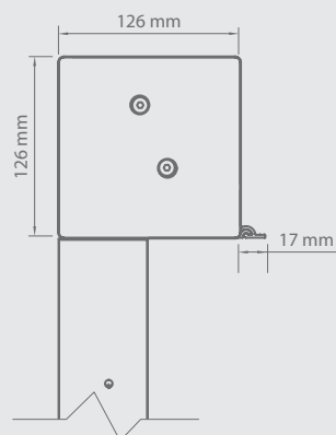
Dimensioni della cassetta
