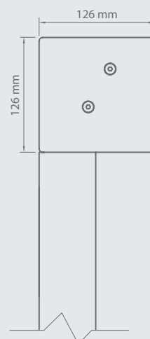
Dimensioni della cassetta
